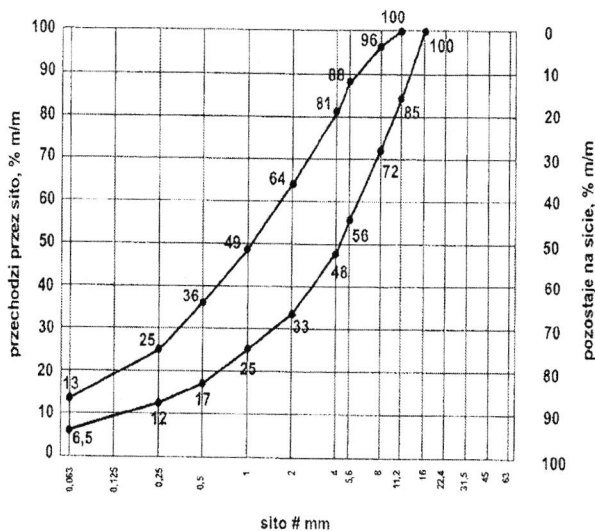
Rys. 4. Krzywe graniczne uziarnienia mieszanki mineralnej 0/11.2 mm
